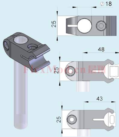
CXGRS 18 Guide Rail Support -Polyamide (护栏夹, 尼龙)
