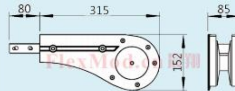
CXBEJ A85 Idler end unit (从动单元)
